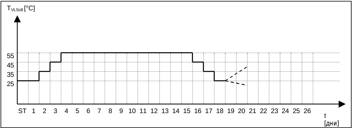
Временной график высушивания цементной стяжки при Belegreifheizen
