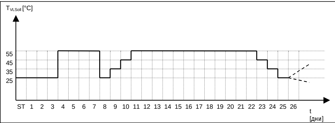
Временной график высушивания цементной стяжки при функциональном и Belegreifheizen
