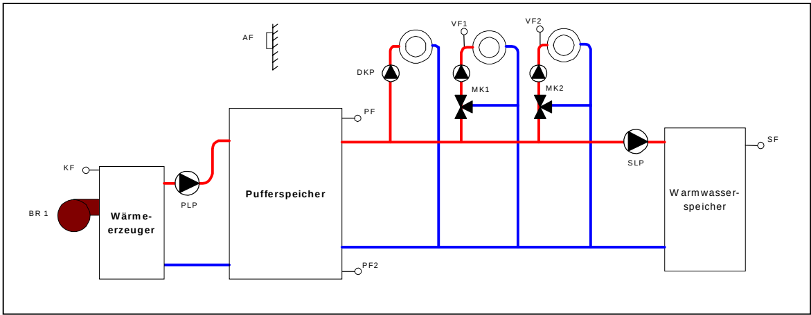
Гидравлическая схема системы отопления:
